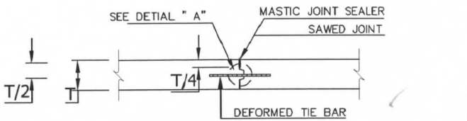
LONGITUDINAL JOINT
