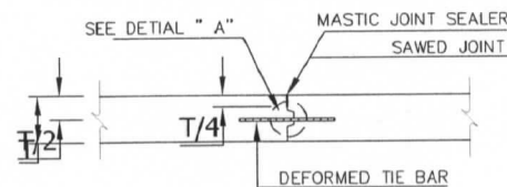
LONGITUDINAL JOINT
