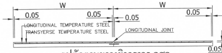
รูปตัดตามขวางผิวจราจร คส.
