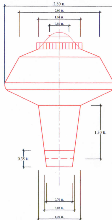
แบบขยายเมนโฮลบนถังแฉมแปยุ มาตราส่วน 1 : 50
