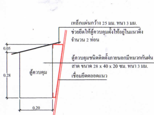
แบบขยายผู้ควบคุม มาตราส่วน 1 : 10
