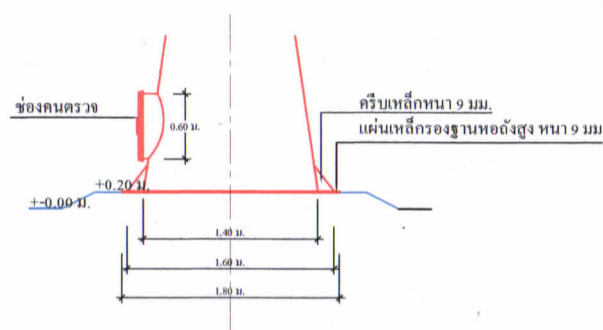
แบบขยายเมนโฮลล่างถังแฉมแปยุ มาตราส่วน 1 : 50
