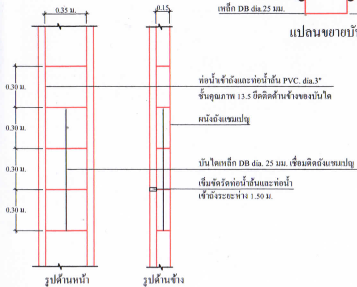
แบบขยายบันได และการยึดท่อน้ำลงและท่อน้ำเข้าถัง มาตราส่วน 1 : 20
