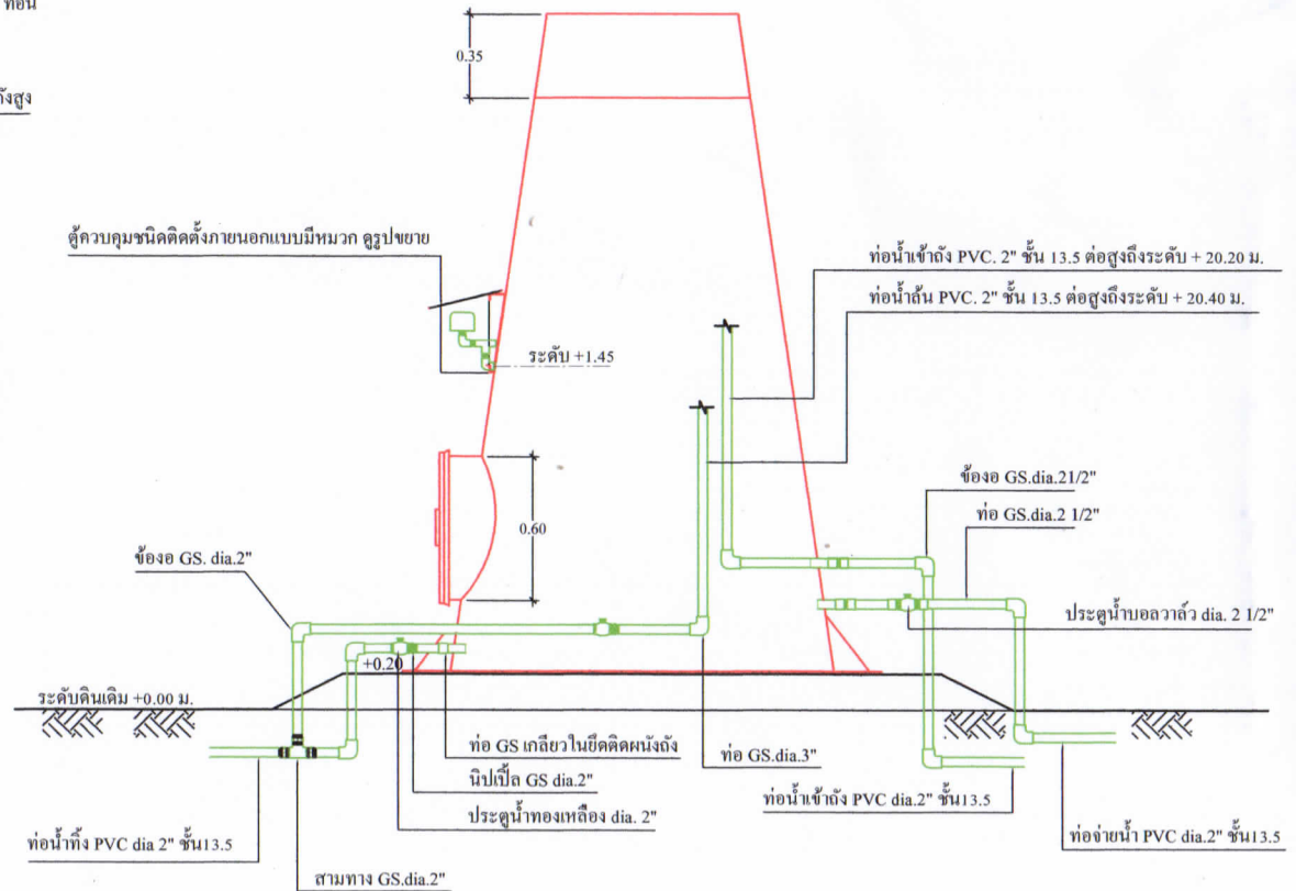
แบบแสดงการเดินท่อในถังแฉกปูน มาตราส่วน 1 : 25
