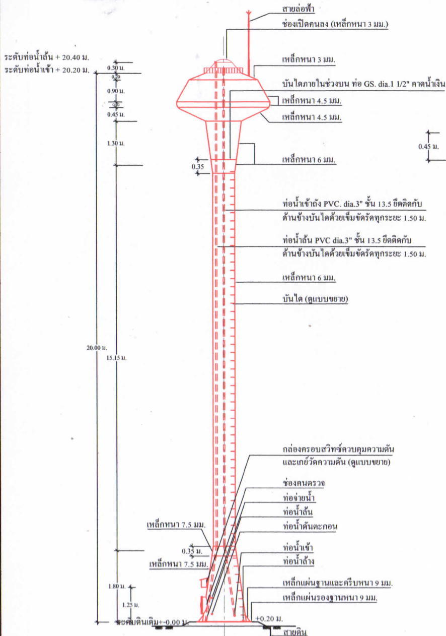
รูปด้านข้างหอดึงสูง แบบดังเหล็กรูปทรงด้วยแฉมแปยุ มาตราส่วน 1 : 100
