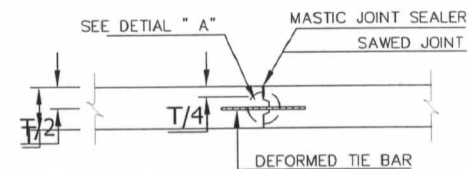
LONGITUDINAL JOINT
