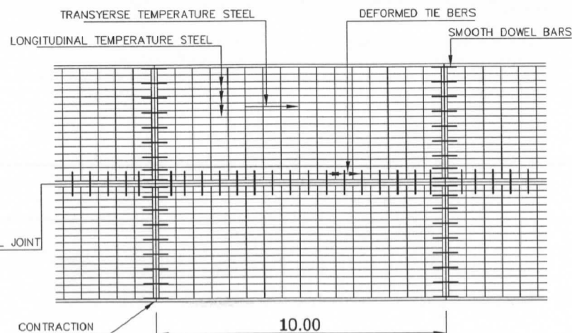
แปลนแสดงการเสริมเหล็กถนน ค.สท.
