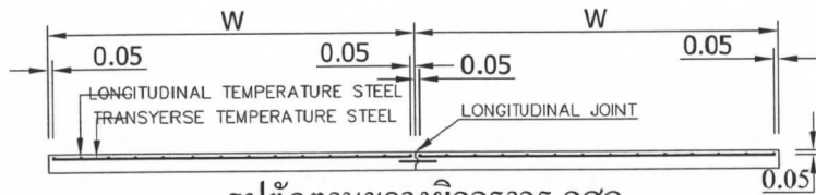
รูปตัดตามขวางผิวจราจร คสท.
